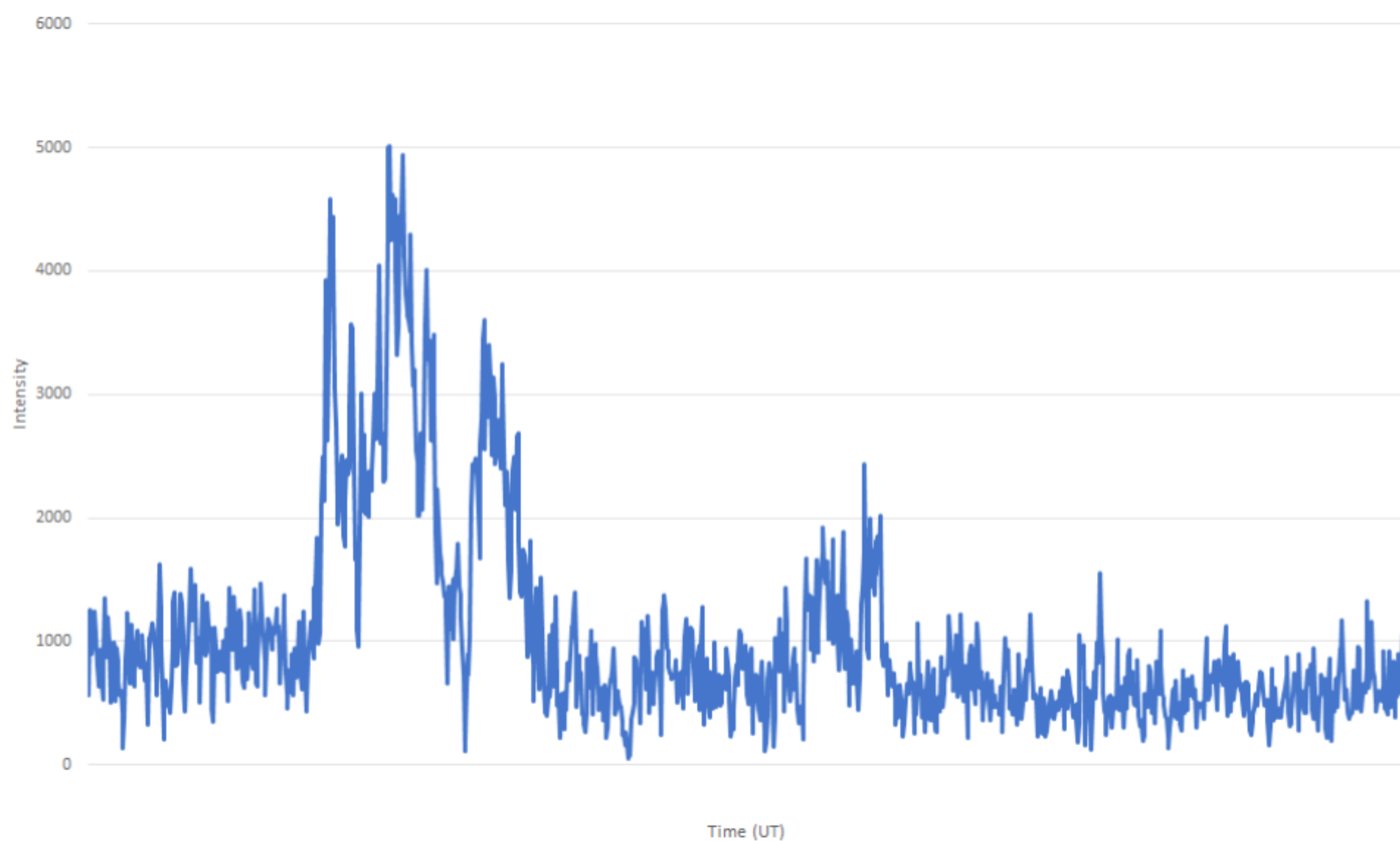
AURORA 20241010_2300 UT-20241011_0200 UT 49.99 MHz Felix Verbelen (Kampenhout/BE)
